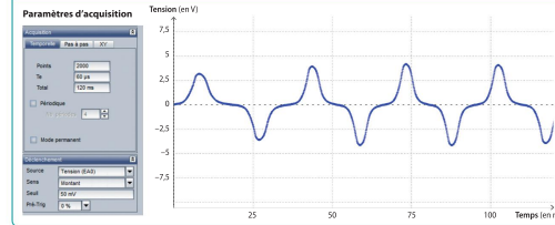
L'interface d'acquisition permet de visualiser sur l'écran de l'ordinateur la tension produite par l'alternateur en fonctionnement.
