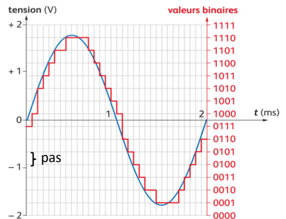
Quantification d'un signal analogique sur 4 bits
