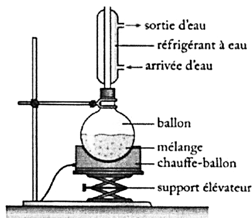
montage à reflux
